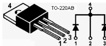
КД641 АС÷ЕС
