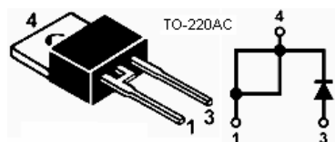
КД641 А÷Е
